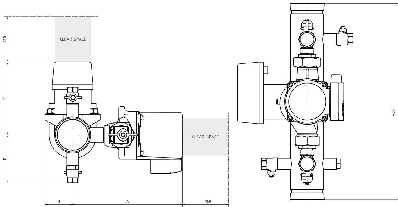
Abb. 1: Zone-Lux® MaBe (mm)
