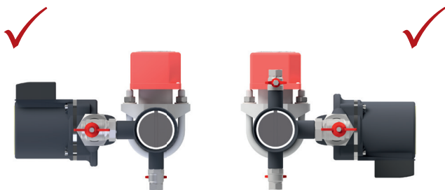
Abb. 2: Zone-Lux® korrekte Ausrichtung
