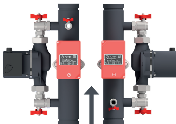
Abb. 4: Zone-Lux® mögliche vertikale Ausrichtung: Pumpe in Strömungsrichtung links
